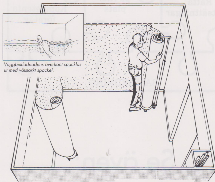
Horisontell väggsättning är enkel med speciellt framtagna hjälpmedel.
